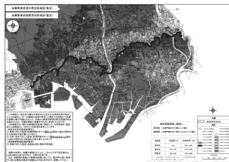
兵庫県津波浸水想定区域図（暫定）は平成23年10月に発表されました。兵庫県HPからダウンロードできます。
